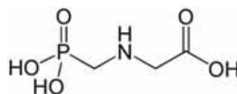
Strukturformel von Glyphosat, Quelle Wikipedia
